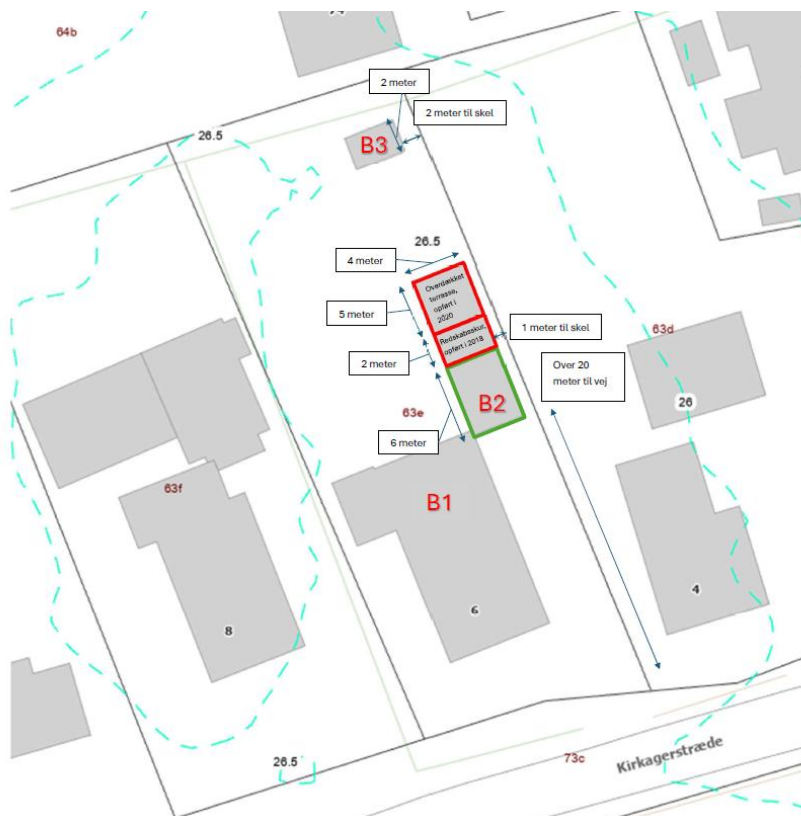
Figur 1: Situationsplan, skur og overdække markeret med rød.
