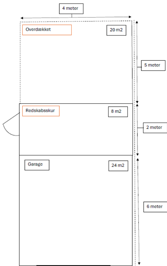
Figur 2: Plantegning
